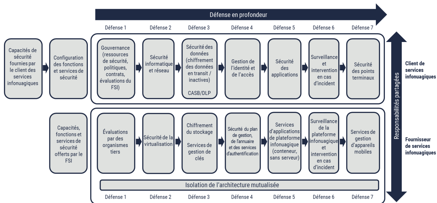
Figure 3 – Concept de la défense en profondeur pour l'infonuagique
